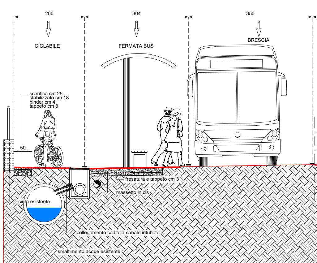
SEZIONE TIPO 1 - LOTTO 1 scala 1:50
